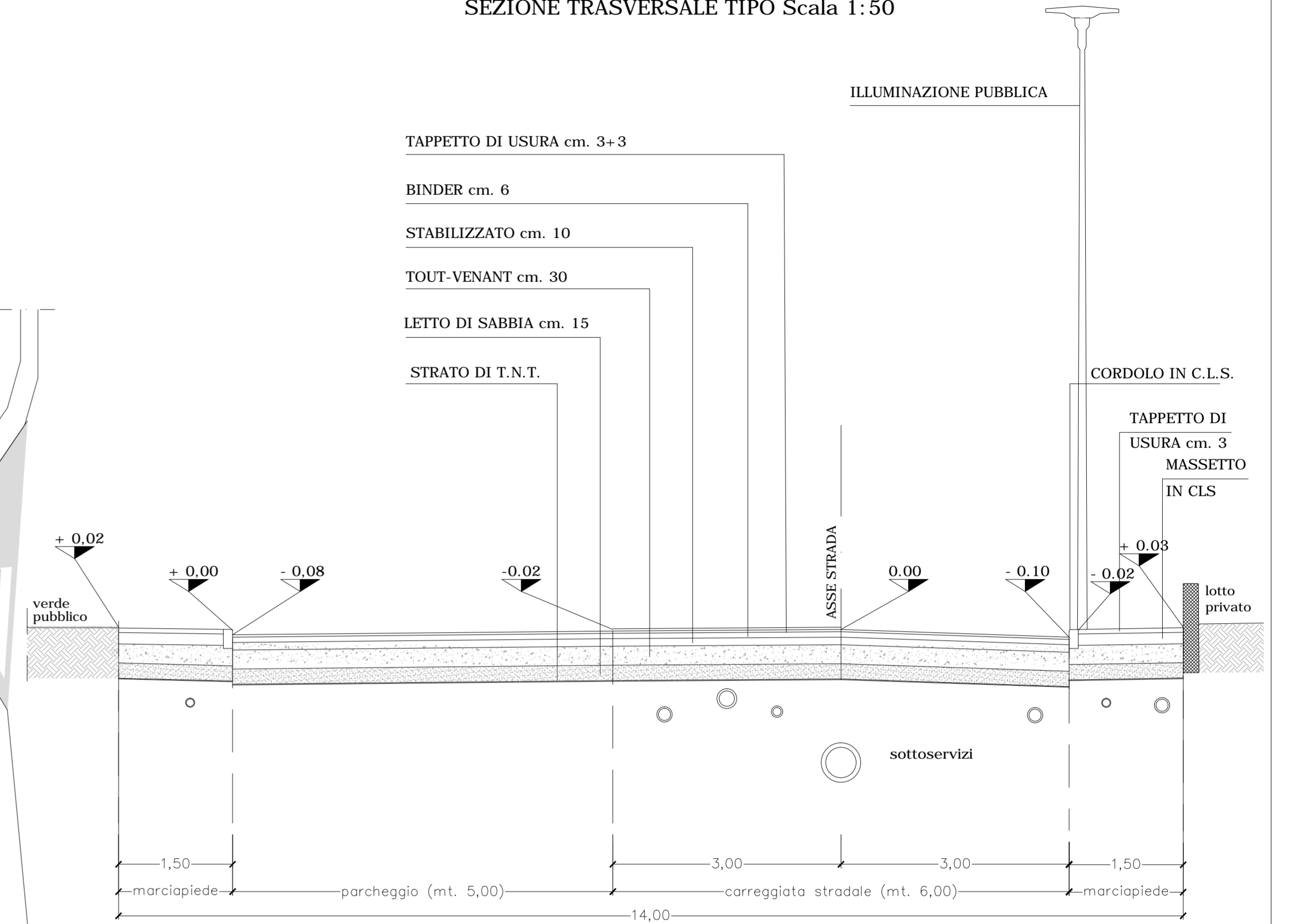
SEZIONE TRASVERSALE TIPO Scala 1:50
